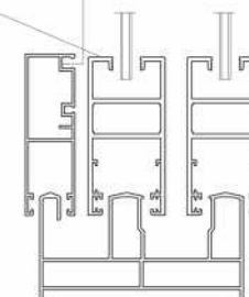
ZJM6102 活动角码配: CCG01 (合和兴)
