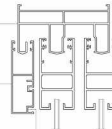
ZJM6130H 角码配: GR6110
